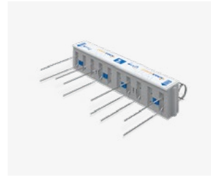
Schöck Isokorb® XT Typ Q-VV positive und negative Querkraft
