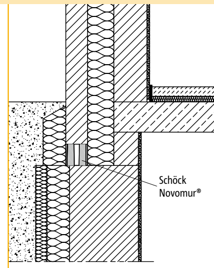
Einbauzustand Schöck Novomur® zweischalig
